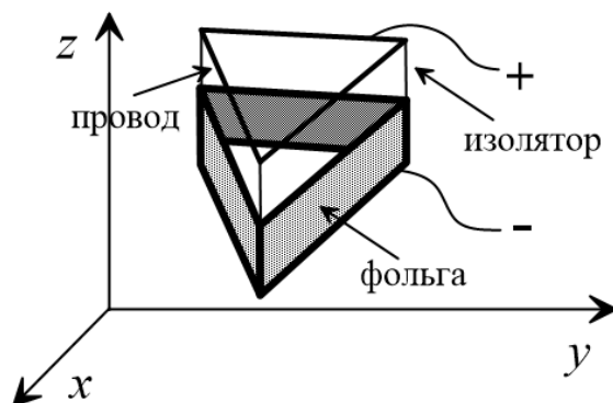
Рис. 23. Лифтер.
