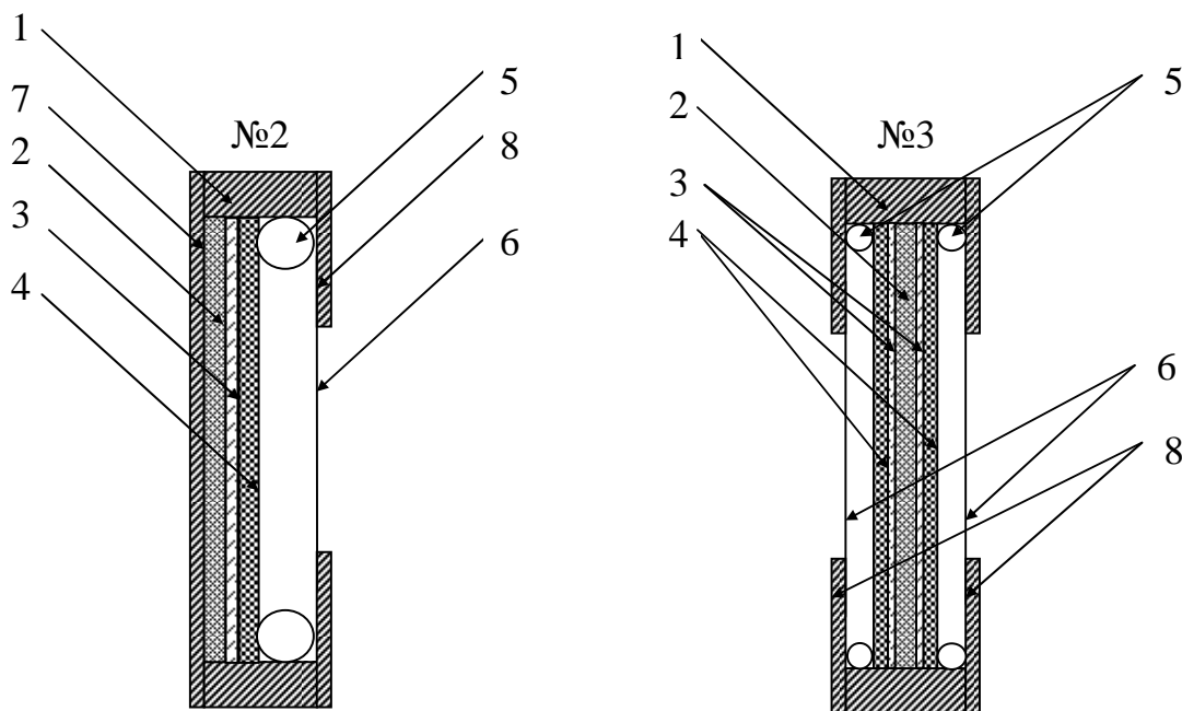
Рис. 114. Тепловые стаканы 2 и 3. В кольцеобразный текстолитовый корпус датчика 1 помещены: нагреватель 2, бронзовая прокладка для выравнивания температурного поля 3, тепломер Герашенко 4, уплотнительное кольцо 5, тонкая изолирующая прокладка 6; датчики закрыты задней крышкой 7 и текстолитовыми кольцами 8. В конструкции №2 используется один тепломер Герашенко, а в конструкции №3 – два тепломера.
