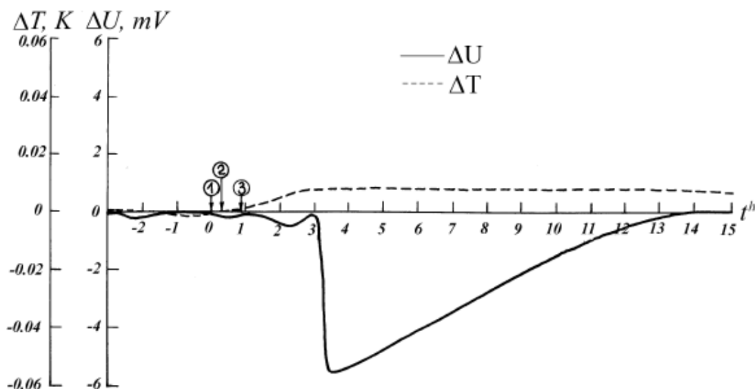
Рис. 79. Пример регистрограммы эксперимента: \Delta U – разностный сигнал детекторов (в милливольтгах), \Delta T – разность внутренних температур детекторов (в градусах), t – время (в часах). 1 – момент включения нагревателя в источнике, 2 – момент закипания, 3 – момент выключения нагревателя в источнике \langle \tau_2 \rangle = (149 \pm 47) мин. Постоянная времени релаксации оценена \sim 360 мин. Время практического окончания эффекта определяется наименее точно. Приблизительно время восстановления (от \Delta U = \Delta U_m до практического окончания эффекта) t_2 оказалось в среднем \langle t_2 \rangle \approx 8 \langle t_1 \rangle , где t_1 – время падения \Delta U ( t_1 = \tau_2 - \tau_1 ).
